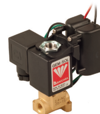
LD032 (GEM-LDO) assembled with A32 (GEM-A) solenoid
