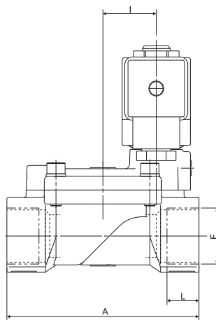
GEM-S-4□r (16 mm orifice)
