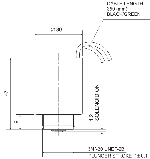
2 Way NC
