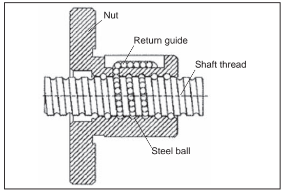
Fig. 11-b Return guide type
