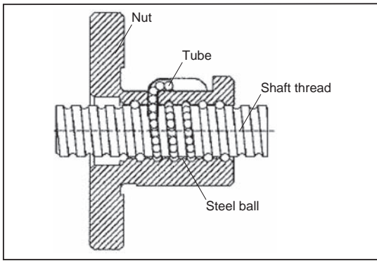
Fig. 11-a Tube type
