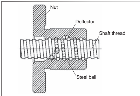
Fig. 12-a Deflector type
